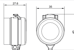
Артикул TS290H Размерный чертёж
