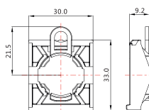
Артикул TS290A Размерный чертёж
