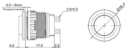
Выпуклая кнопка с короткими контактами
