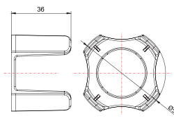
Артикул TS290P Размерный чертёж
