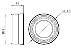
Артикул TS290E Размерный чертёж
