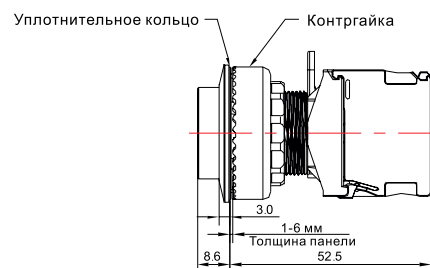
Утопленный выпуклый тип
