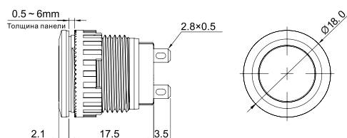
Плоская кнопка с короткими контактами
