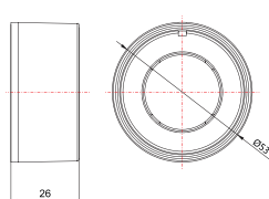
Артикул TS290N Размерный чертёж
