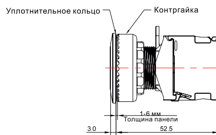
Утопленный плоский тип
