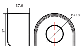
Артикул TS290G Размерный чертёж
