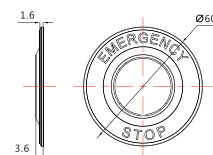
Артикул TS290D Размерный чертёж
